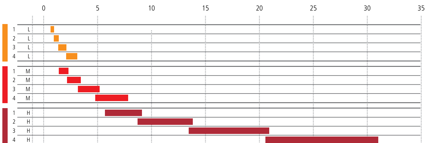
VELOCITÀ DI AVANZAMENTO IN KM/H DEL CAMBIO MECCANICO 12+12
